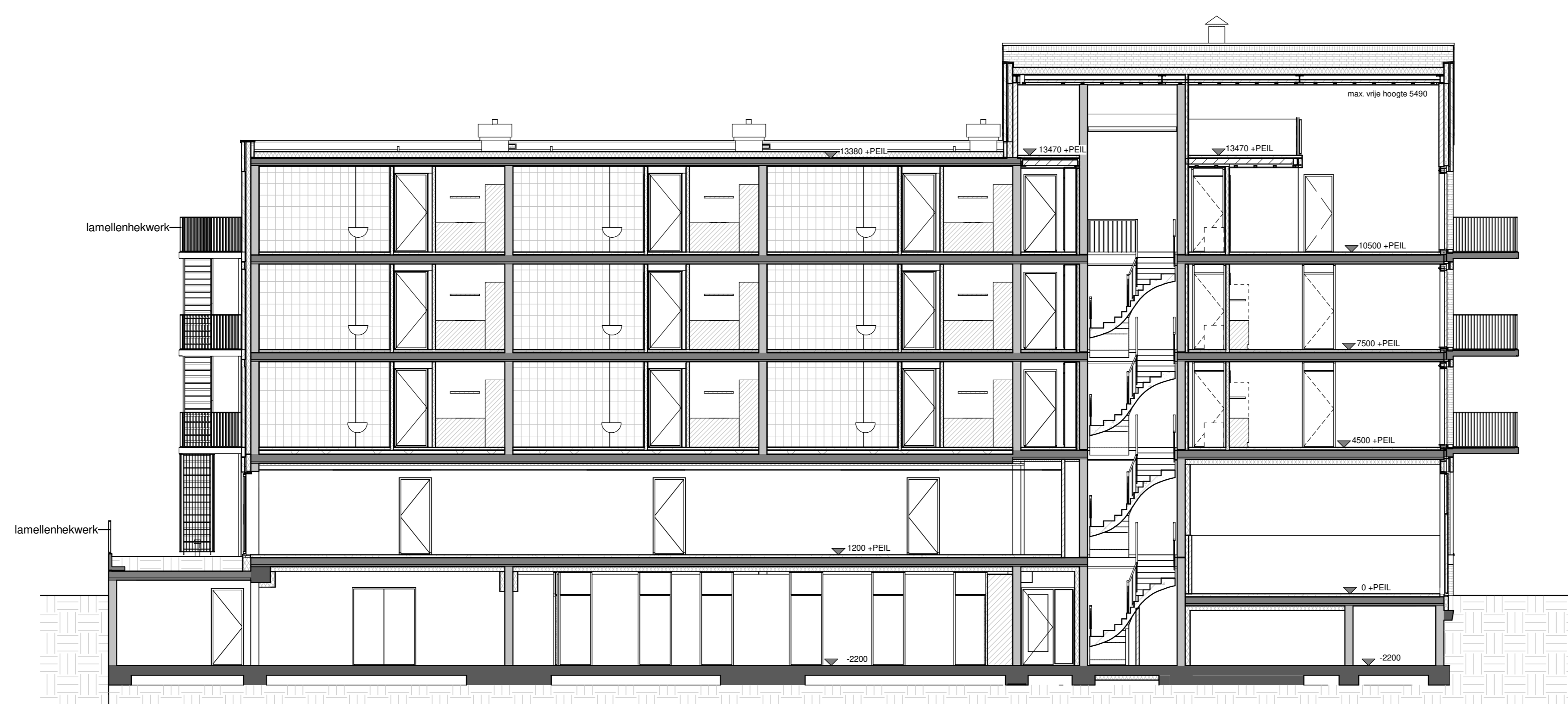
doorsnede B4-B
