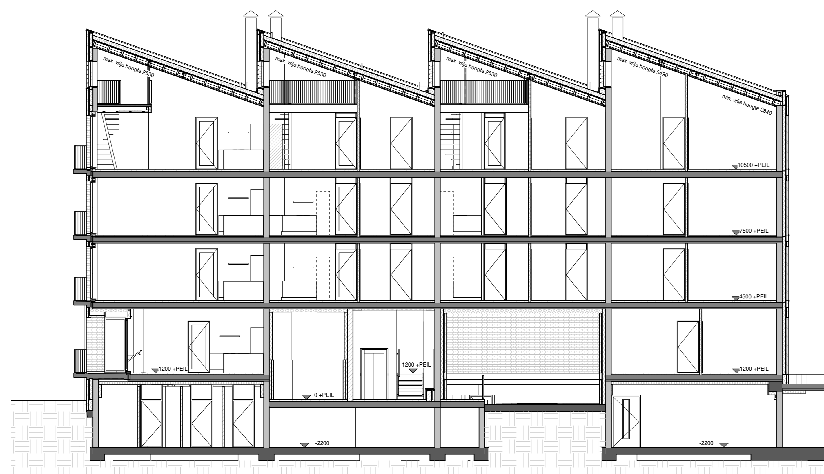
doorsnede B4-A
